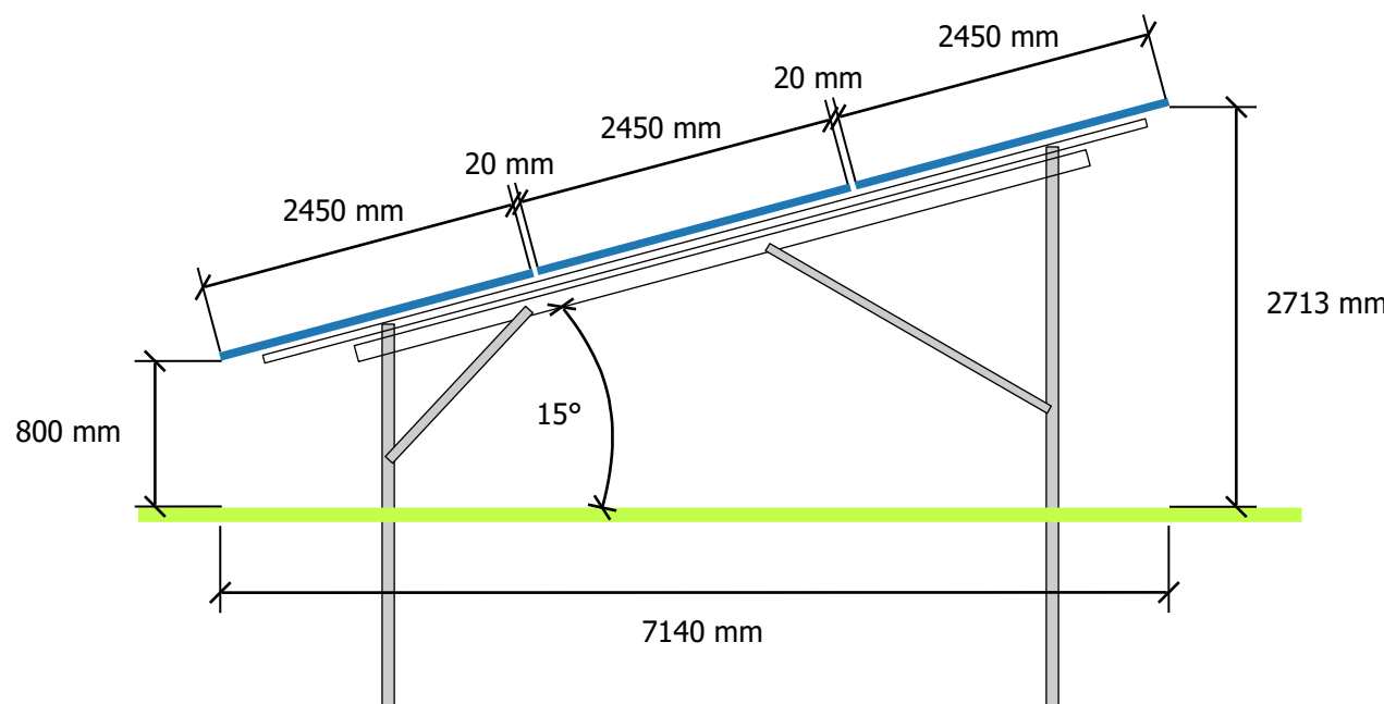
Schnittzeichnung Modultisch
